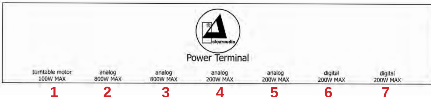
Abb. 2: Erläuterung der Anschlüsse
